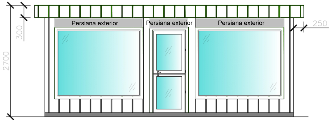
ELEVACIÓN SUR
